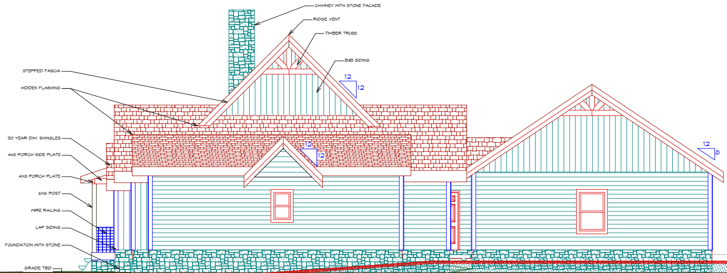
RIGHT ELEVATION
